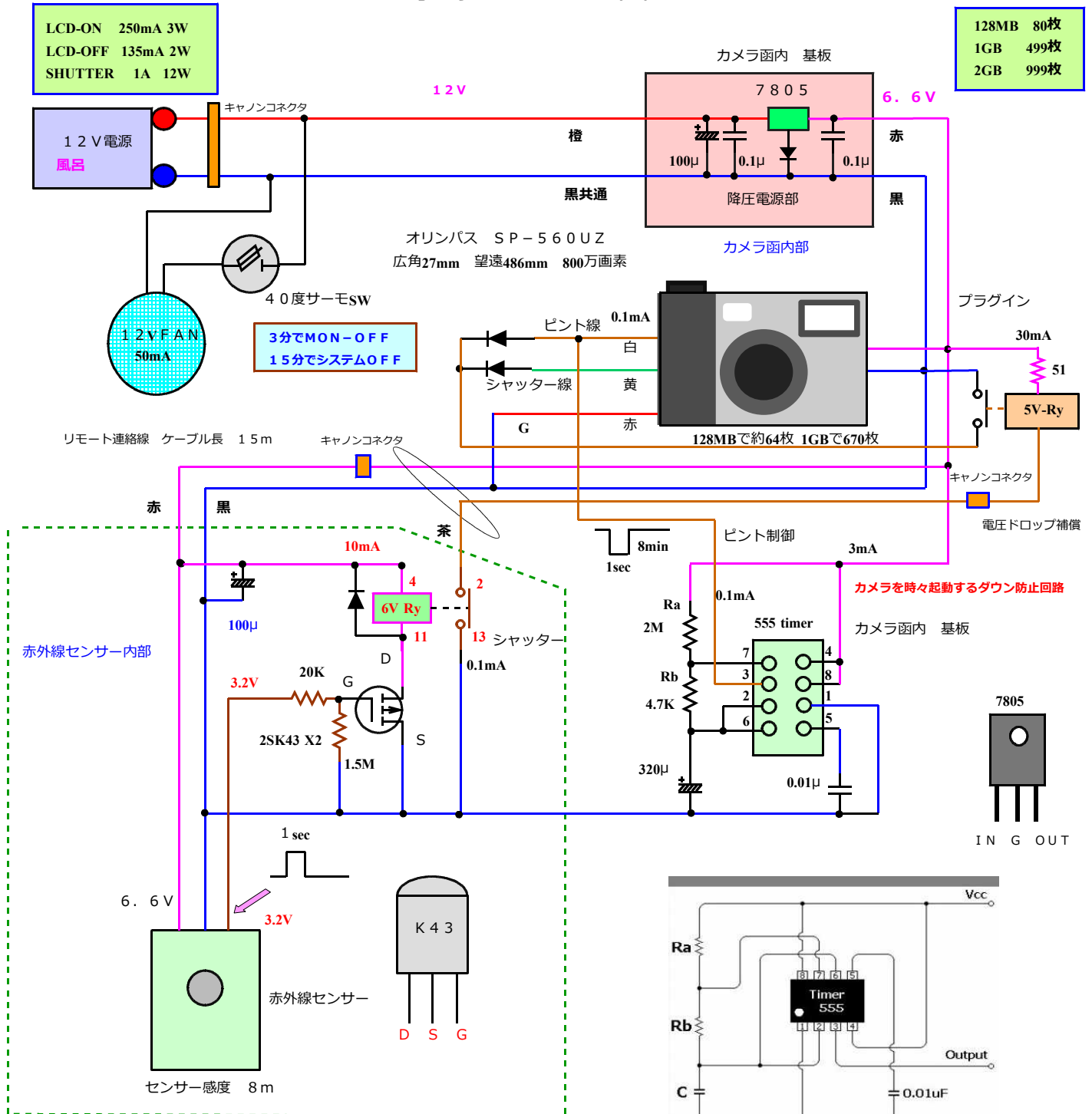
555自走基本接続図
