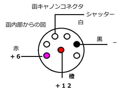
555自走基本接続図
